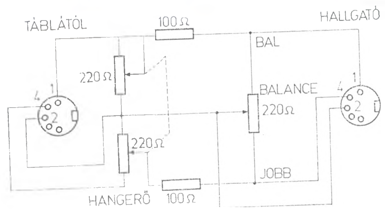
LEHALLGATÓ CSATLAKOZÓ TÁBLA
